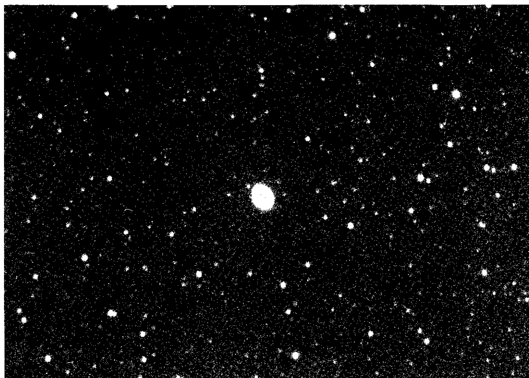
こと座M57リング星雲
