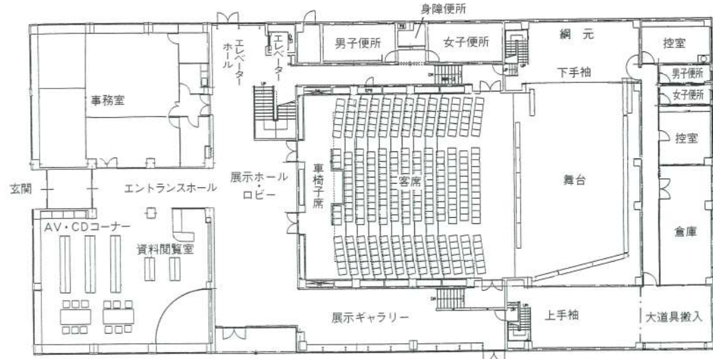
1階の平面図
