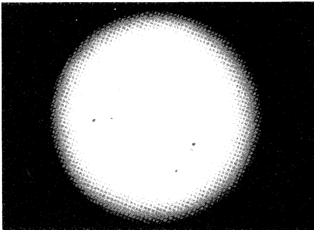
黒く見えるが、温度は4000度もある太陽の黒点
