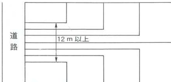
① 道路位置指定を用いない開発計画例
