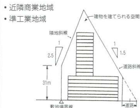
図 2. 隣地境界、道路境界からの斜線制限
