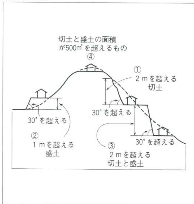
図2. 宅地造成
