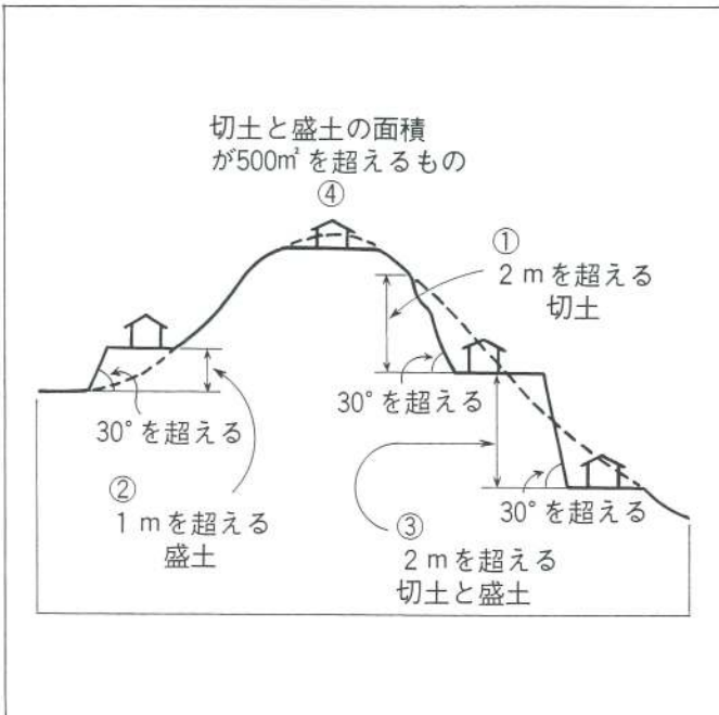
図2. 宅地造成
